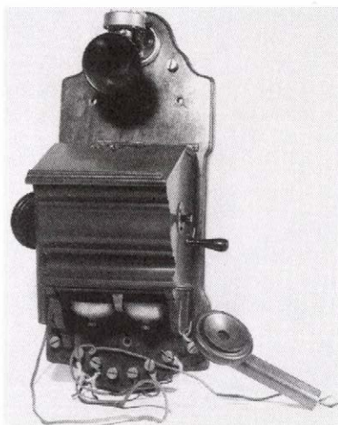
LB 1 fali távbeszélő-készülék
