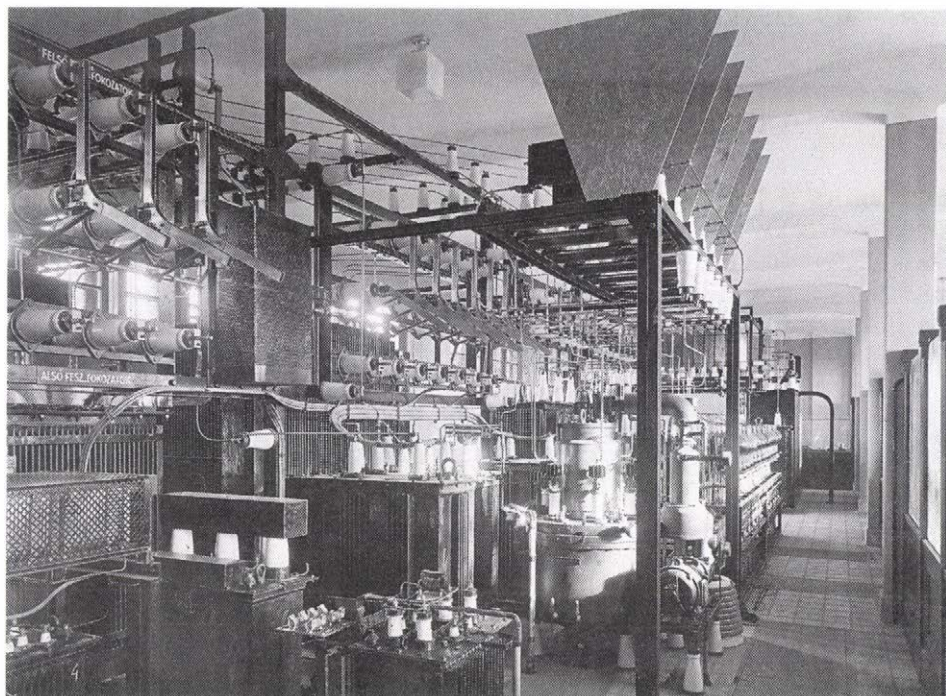
A 120 kW-os adó Lakihegyen
