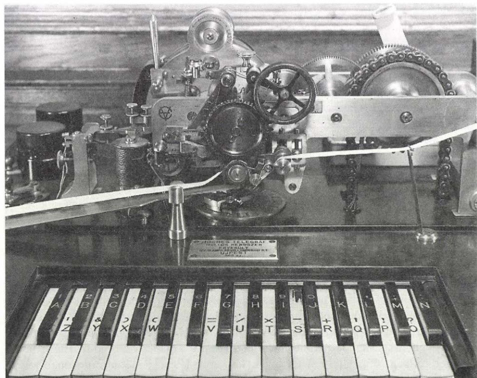
Hughes típusú távíró: billentyűzet, adó-, vevő-, nyomtató- és meghajtószerkezet
