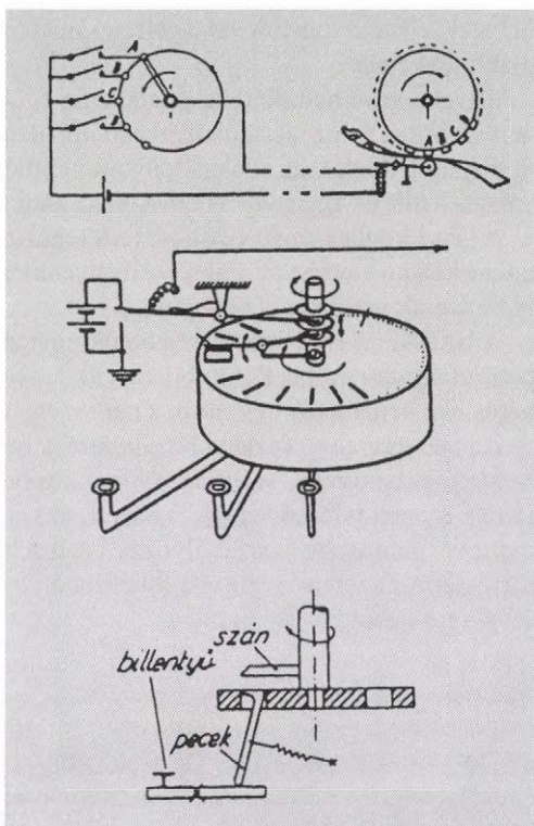
A Hughes típusú távirógép működési elve
