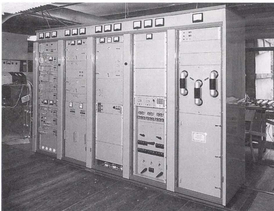
10/2 kW-os I. sávi televízióadó (ORF Jauerling)
