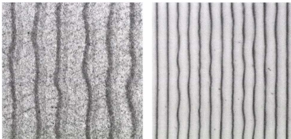
Normál és mikrobarázdás hanglemez, hangbarázdái azonos nagyításban
