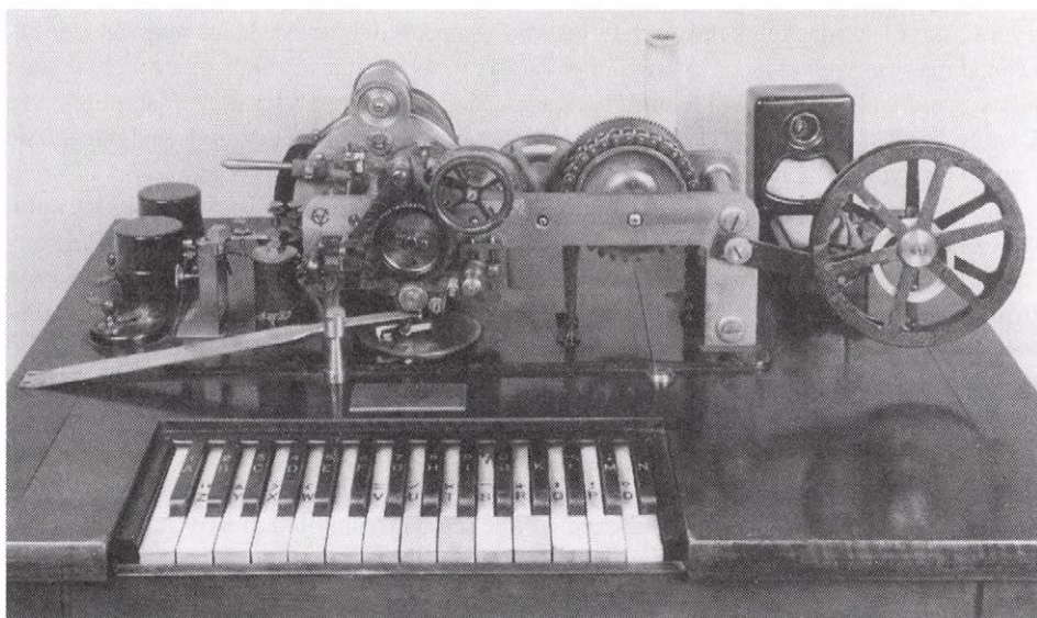
Hughes-féle betűnyomó táviró
