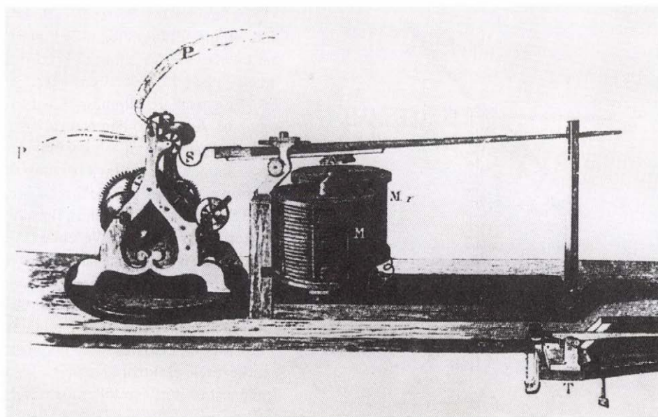
Morse-féle távíró, 1844
