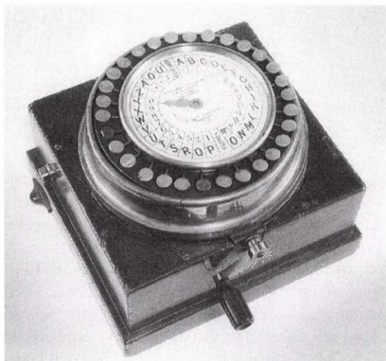
Mutatólapos távjelző
