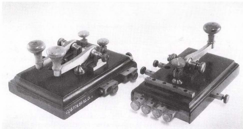
Kettős billentő és egyes billentő telepváltóval
