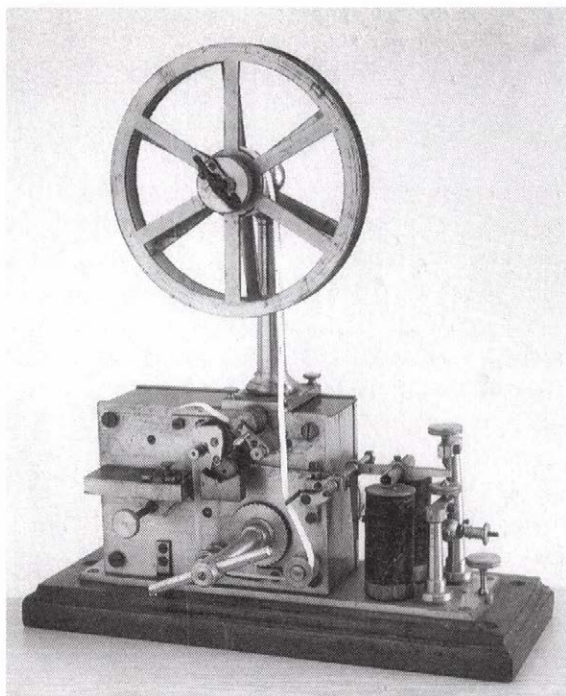
Siemens-féle kékíró
