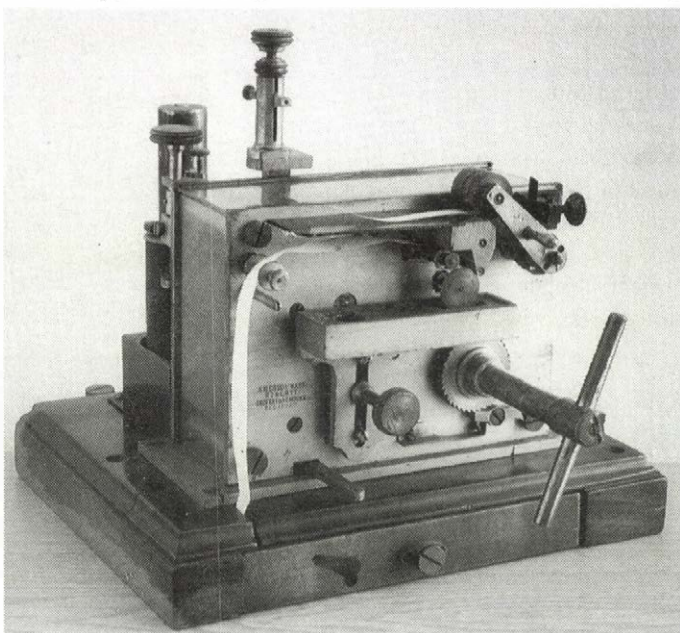
Hollós-féle kékíró
